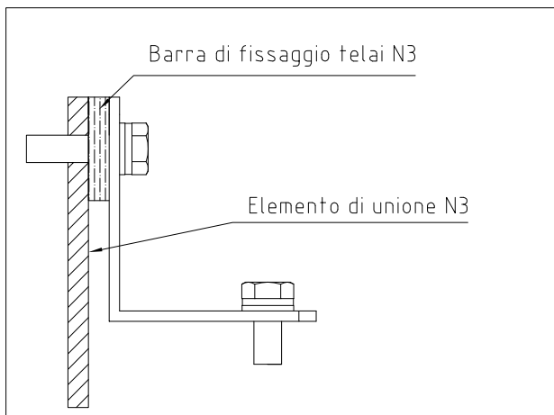
Esempio di ancoraggio sotto struttura di un telaio N63E: La staffa non interferisce con l'installazione di un telaio N3 schienato con l'apposito elemento di unione
