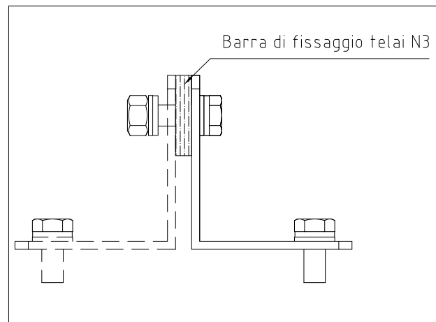
Esempio di ancoraggio sotto struttura di due telai N63E: La seconda staffa (tratteggiata) va fissata tramite dado e rondelle M8 fornite a corredo
