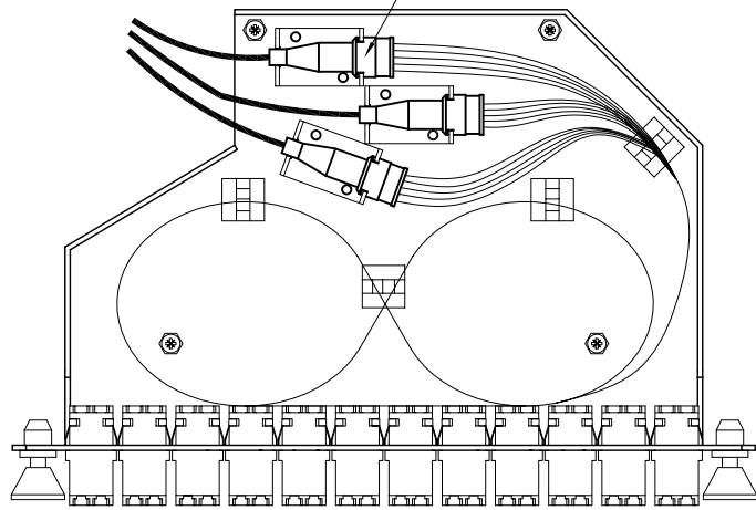
Esempio percorso fibra
