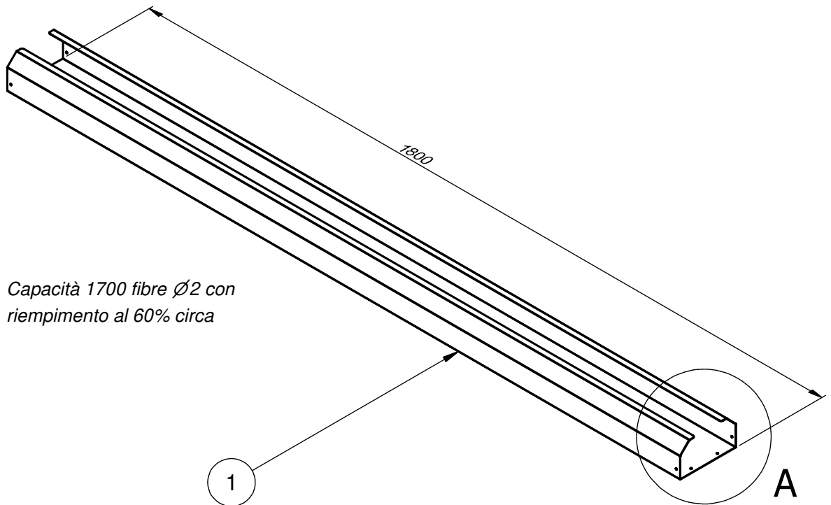
Dett. A
